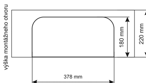
BOČNÝ POHĽAD NA MONTÁŽNY OTVOR
