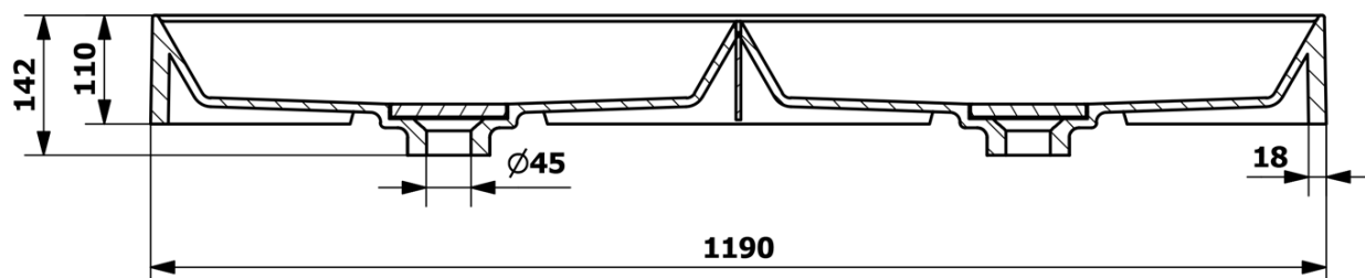
C-C ( 1:6 )
