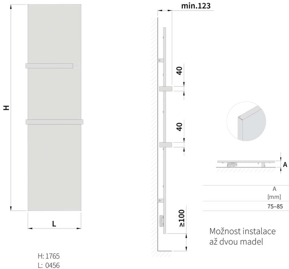
Madlo jednostranné
