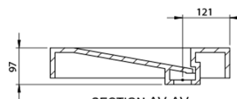
SECTION AV-AV
