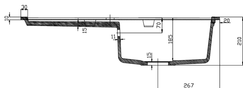
REZ A-A
