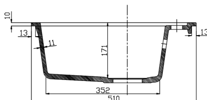
REZ B-B
