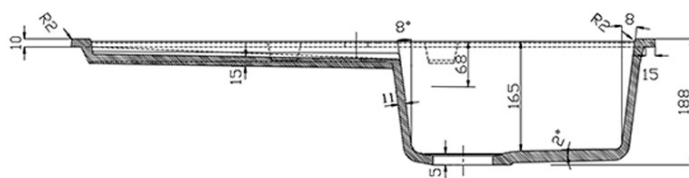
REZ A-A
