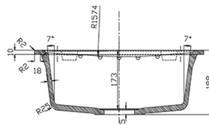
REZ B-B
