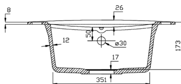
REZ B-B
