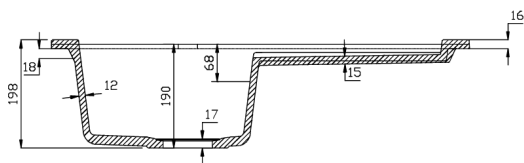
REZ A-A
