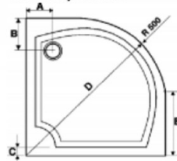
Technický náčrt
