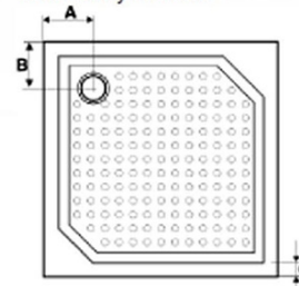
Technický náčrt
