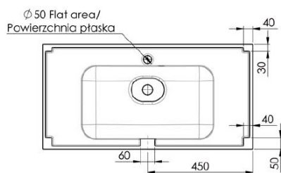
Bottom view/ Widok od dołu
