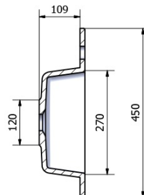
B-B ( 1 : 6 )
