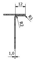
A-A (1 : 1)
