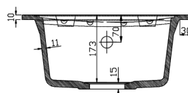
REZ B-B
