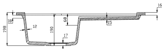
REZ A-A
