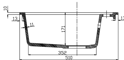
REZ B-B
