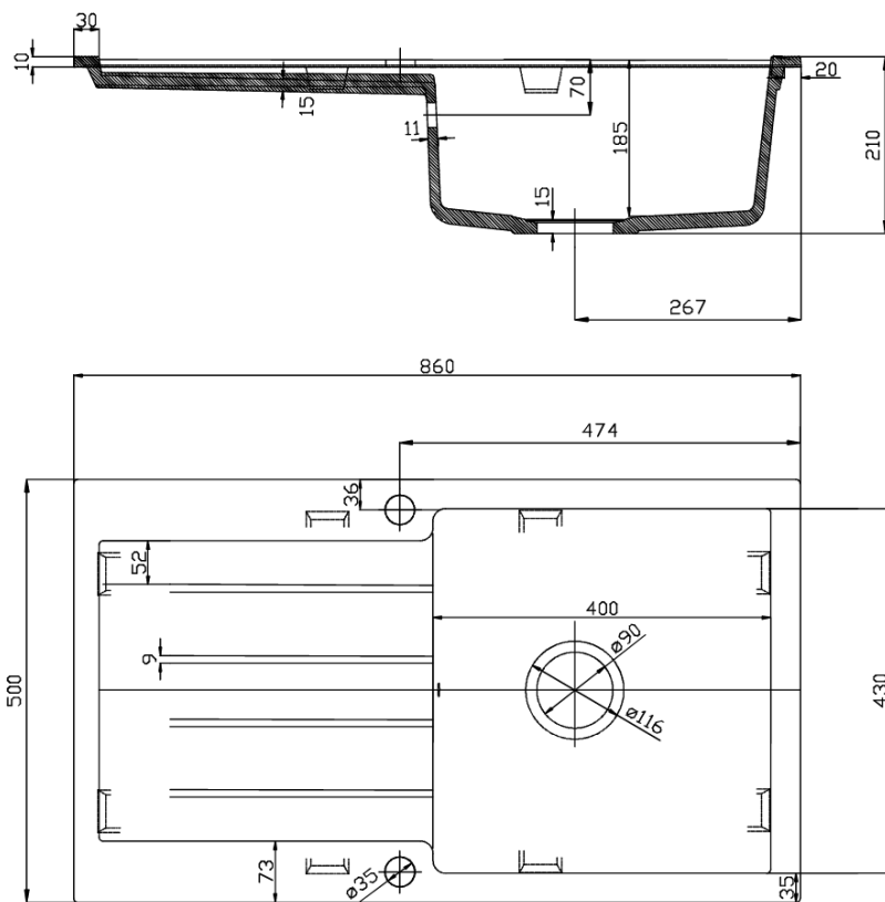
REZ A-A
