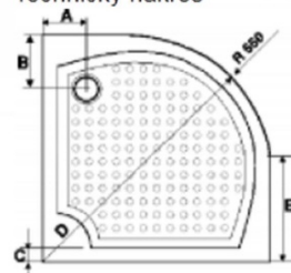
Technický náčrtek
