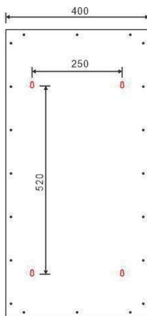
Hátulról
