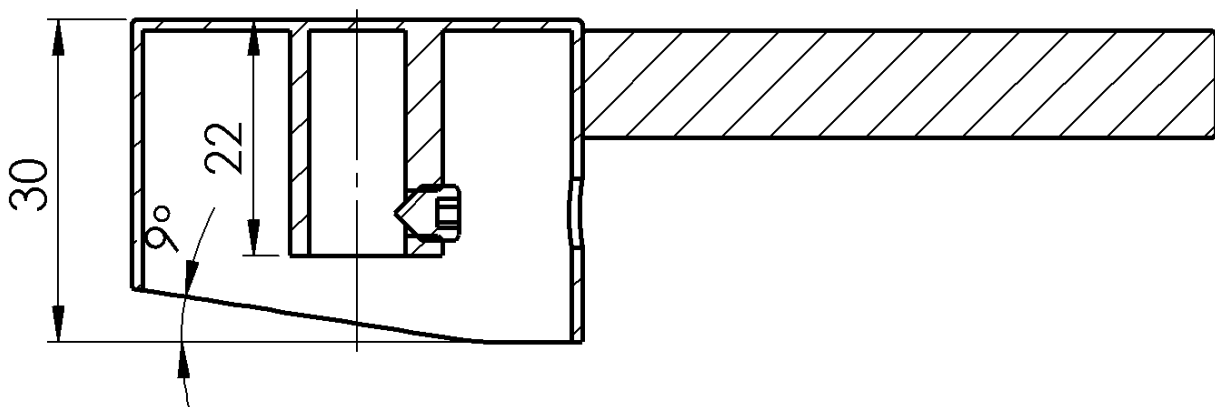
ŘEZ A-A
