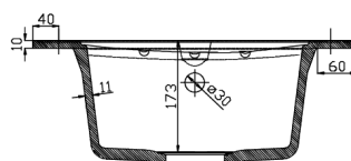
REZ B-B
