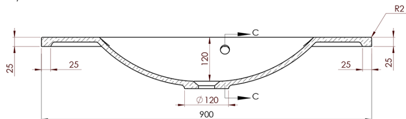
A-A (1:5)
