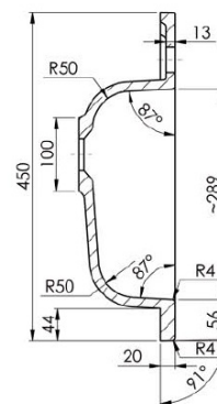
B-B (1 : 5)
