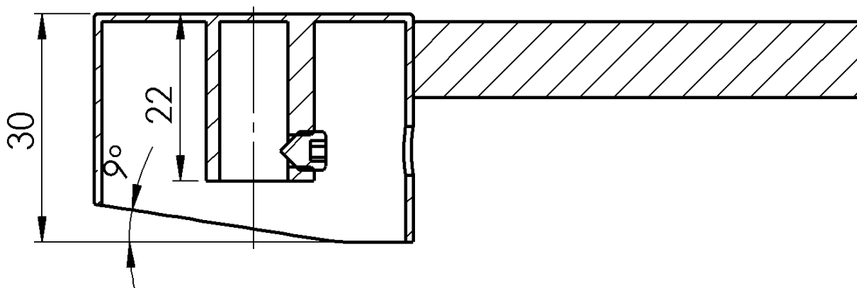
ŘEZ A-A
