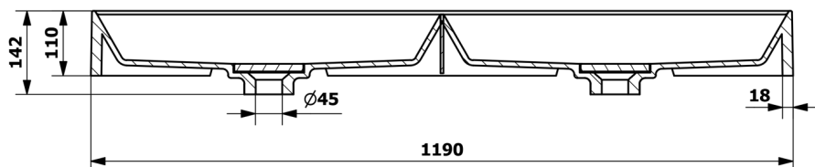
C-C ( 1:6 )
