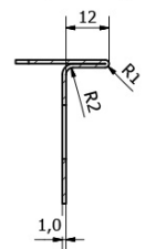
A-A (1 : 1)
