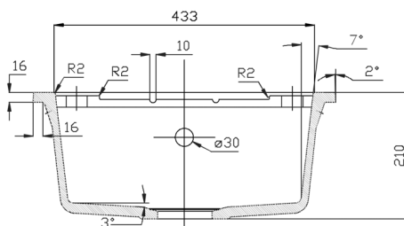
REZ B-B
