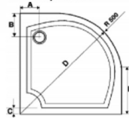
Technický náčrtek
