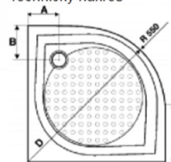
Technický náčrtek
