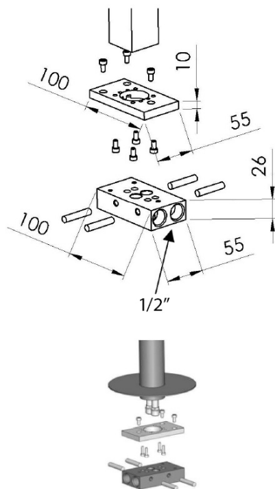
FISSAGGIO FIXING DEVICE
