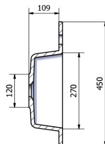
B-B ( 1 : 6 )
