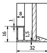
A-A ( 1 : 1 )
