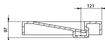
SECTION AV-AV
