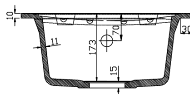
REZ B-B
