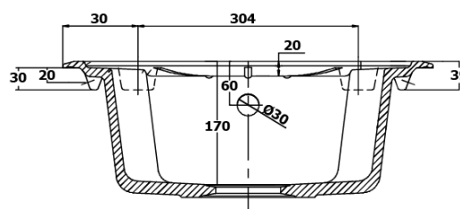
REZ B-B
