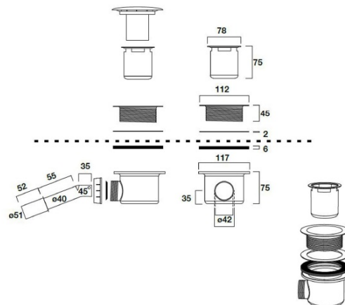
9056 Piletta sifonata per piatti doccia foro Ø 90 Shower tray drain plug Ø 90
