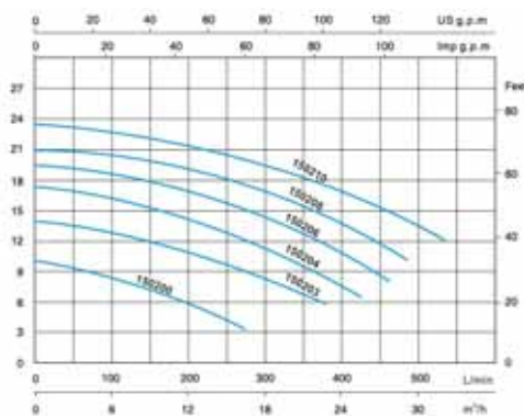
Charakteristika čerpadel/Pump curve
