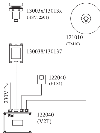
2 122040 V2T elektronika v zapojení pro spínání halogenového osvětlení ovládaná tlačítkem TM10. 122040 V2T control electronics wired for halogen light switching controlled with TM10 button.
