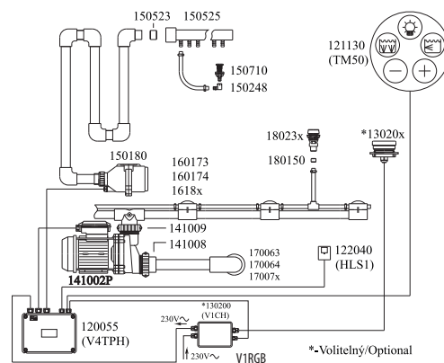
18 120055 V4TPH elektronika v zapojení pro spínání čerpadla a kompresoru s pulsací, regulací otáček kompresoru, chromoterapií (13020x+V1RGB nebo 130210), jističím proti chodu naprázdno hladinovým snímačem HLS1 a možnosti automatického vysoušení. 120055 V4TPH control electronics wired for pump and blower switching with pulsation, blower speed regulation, chromotherapy (13020x+V1RGB or 130210), water level sensor HLS1 for dry run protection and pos. automatic drying.
