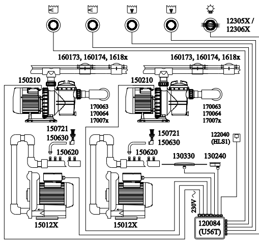
13 120084 elektronika U56T ovládaná piezo a mikrozdvihovými tlačítky 120084 control electronic U56T controlled with piezo and micro-lifting buttons
