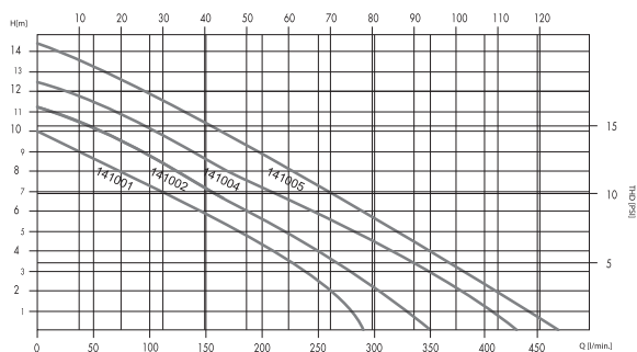
Charakteristika čerpadel/Pump curve
