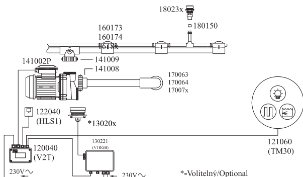
5 120040 V2T elektronika v zapojení pro spínání čerpadla s jistištěm proti chodu naprázdno hladinovým snímačem HLS1. 120040 V2T control electronics wired for pump switching with HLS1 water level sensor for dry run protection.
