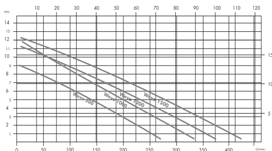
Charakteristika čerpadel/Pump curve
