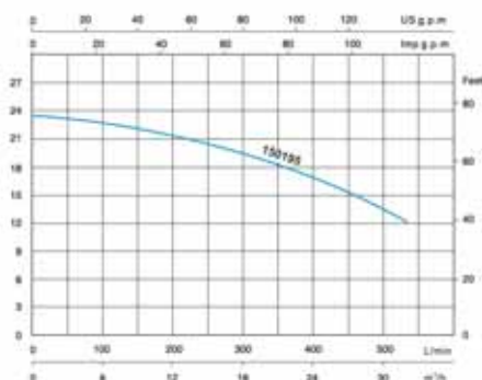
Charakteristika čerpadel/Pump curve
