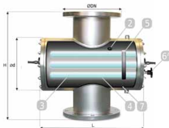
2 - Teplotní senzor/Temperature sensor 3 - UVM lampa/UVM® lamp 4 - Křemenné pouzdro /Quartz sleeve 5 - Pohon stěrače/Wiper mechanism 6 A – Ruční stěrač/Manual wiper 7 - Komora UV lampy z nerezové oceli 316L s leštěným vnitřním povrchem/ 316L stainless steel UV reactor with polished internal surface
