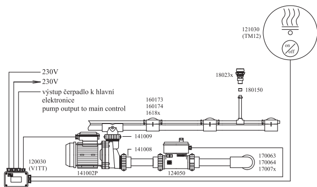
3 120030 V1TT elektronika pro nezávislé spínání topení. 120030 V1TT control electronics for independent switching of heating
