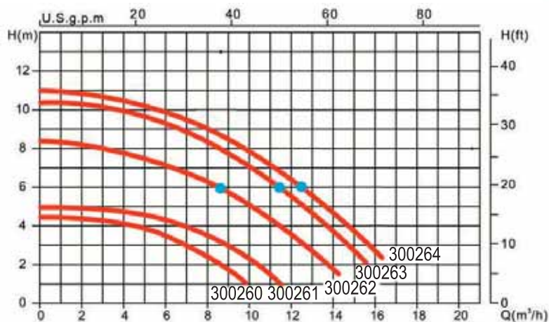
Charakteristika čerpadel/Pump curve
