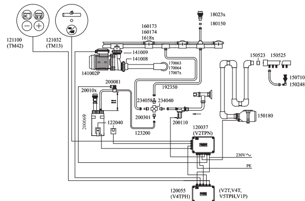
4 120055 V4TPH elektronika v zapojení pro řízení vzduchové a vodní masáže s desinfekčním proplachem STREAMCLEAN řízeným elektronikou 120037 V2TPN. Elektronika V2TPN může být kombinována s většinou hlavních řídicích elektronik. 120055 V4TPH electronics wired for air and whirlpool control with STREAMCLEAN flush disinfection controlled by the 120037 V2TPN electronics. The V2TPN electronics can be combined with most of the main control electronics.
