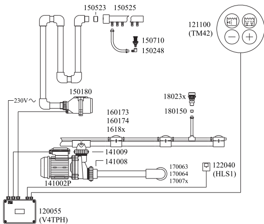
15 120055 V4TPH elektronika v zapojení pro spínání s pulsací čerpadla a kompresoru a s regulací otáček kompresoru vč. jističím proti chodu naprázdno hladinovým snímačem HLS1 a možnosti automatického vysoušení. 120055 V4TPH control electronics wired for pump and blower switching with pulsation and blower speed regulation incl. water level sensor HLS1 for dry run protection and pos. automatic drying.
