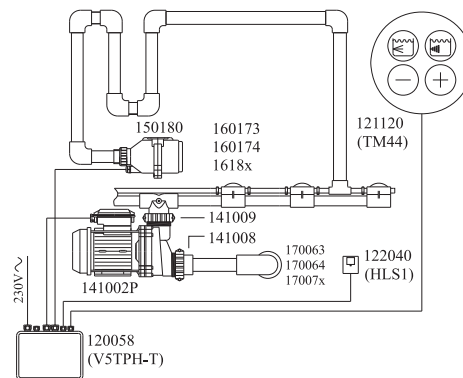
16 120058 V5TPH-T elektronika v zapojení pro spínání čerpadla s pulsací a turbo funkcí vč. regulace otáček kompresoru připojeným do rozvodu vodní masáže pro výrazné zvýšení masážního efektu, vč. jističím proti chodu naprázdno hladinovým snímačem HLS1. 120058 V5TPH-T control electronics wired for pump with pulsation and blower turbo function incl. blower speed control connected to the whirlpool pipes for extra massage power, incl. water level sensor HLS1 for dry run protection.
