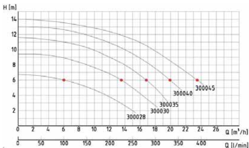
Charakteristika čerpadel/Pump curve
