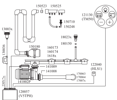
17 120057 V5TPH elektronika v zapojení pro spínání čerpadla a kompresoru s pulsací, regulací otáček kompresoru, osvětlením (halogen nebo LED CoolLight), jističím proti chodu naprázdno hladinovým snímačem HLS1 a možnosti automatického vysoušení. 120057 V5TPH control electronics wired for pump and blower switching with pulsation, blower speed control, light (halogen or LED CoolLight), water level sensor HLS1 for dry run protection and pos. automatic drying.
