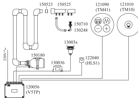
14 120056 V5TP elektronika v zapojení pro spínání kompresoru s pulsací a regulací otáček a chromoterapie (130210 nebo 130200+V1CH) vč. hladinového snímače HLS1 a možnosti automatického vysoušení. 120056 V5TP control electronics wired for blower switching with pulsation and speed regulation and chromotherapy (130210 or 130200+V1CH) incl. water level sensor HLS1 for dry run protection and pos. automatic drying.
