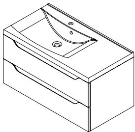
50093 LUCIOLA 90 x 48 cm 89,7 x 45 x 47,8 cm WA092-XXXX
