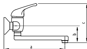
Rozměry a/b/c
