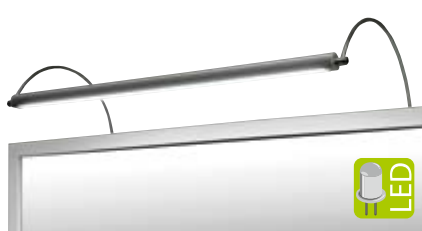
FROMT LED 12 V, 5500 K, IP67, aluminium ED847 7 W, długość 470 mm, 510 lm 285,00 ED877 12 W, długość 770 mm, 860 lm 343,00 ED899 15 W, długość 1020 mm, 1100 lm 393,00
